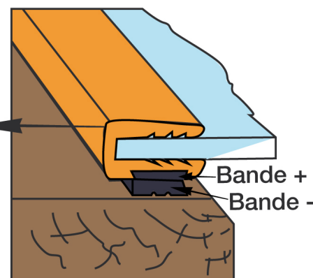
Profil encadrement en PVC sur les trois côtés.
