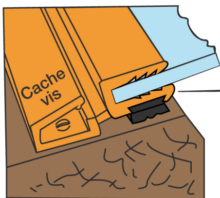
Profil à charnière PVC co-extrudée fixé par vis cachées sur un côté.
